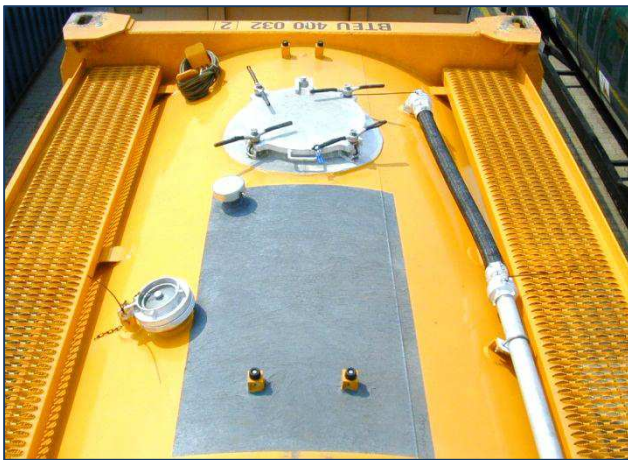
Dachansicht mit Laufgitter und Anti-Rutsch-Belag
